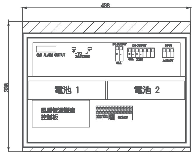
後視圖
